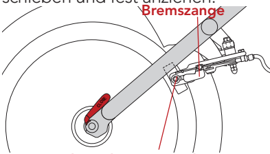
An der Felge ausgerichteter Bremsklotz
